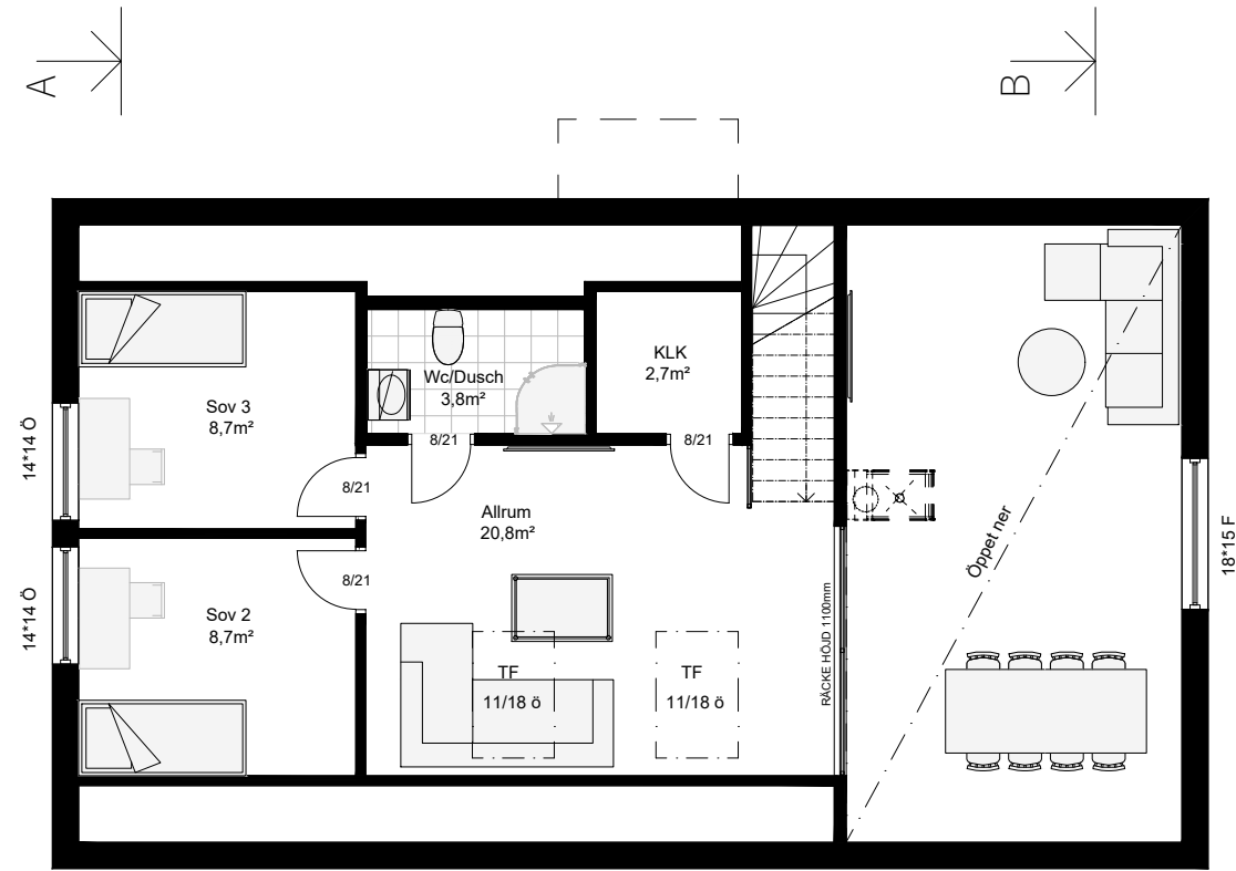
VINDSPLAN MED RYGGÅS-STANDARD
