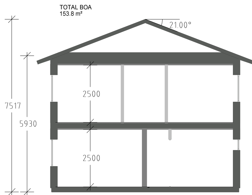
SEKTION
