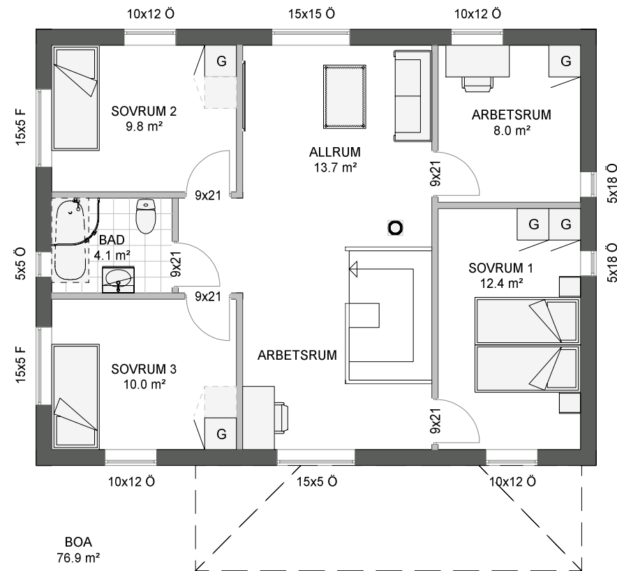
ÖVRE PLAN
